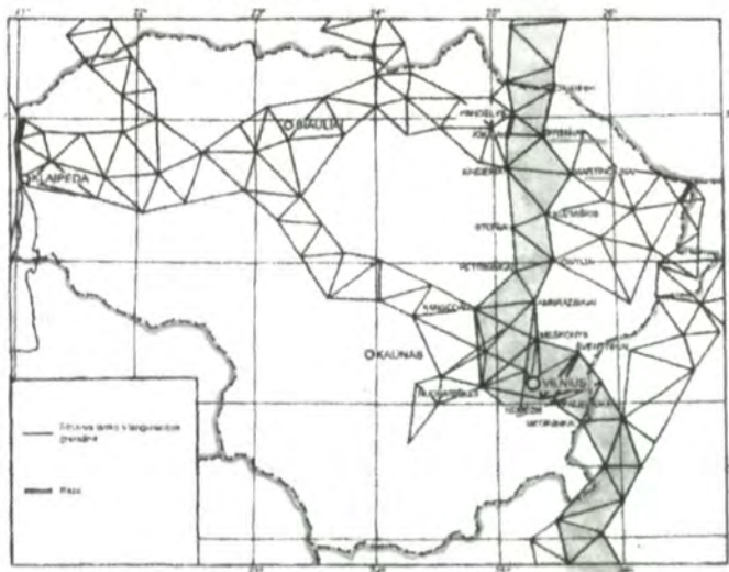
9 pav. K. Tennerio sudarytas trianguliacinių matavimų tinklas, panaudotas Struvės geodeziniam lankui, kerta Lietuvą
