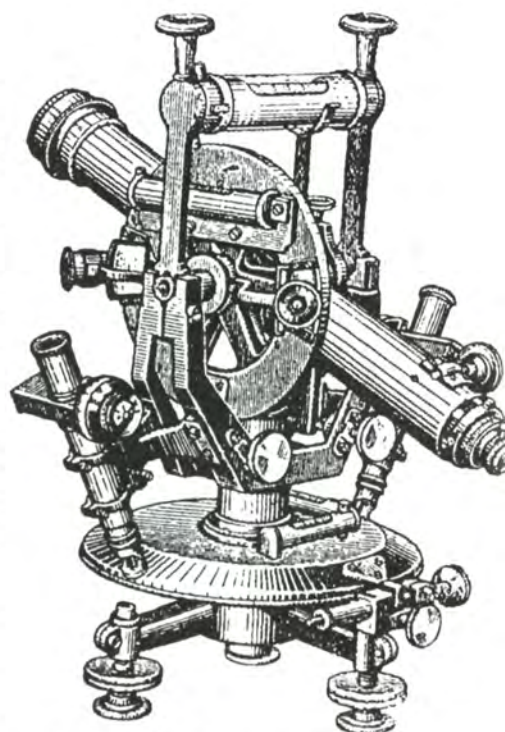
17 pav. Struvės laikų teodolitas
